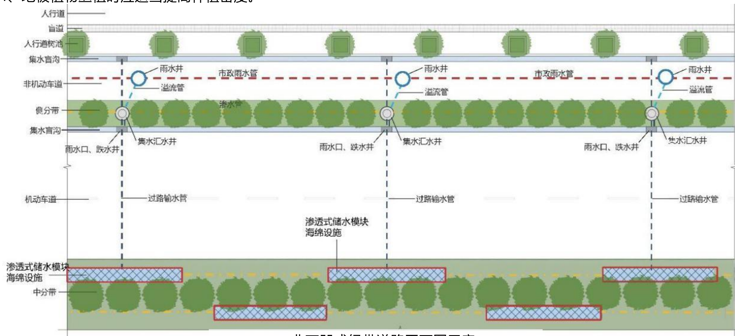
非下凹式绿带道路平面图示意
